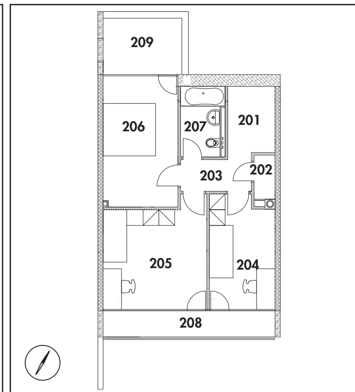
2. NP Půdorys ▼
